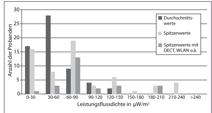
Abb. 1: Einteilung der Probanden nach Messwerten für den Durchschnitts- bzw. Spitzenwert der GSM-Leistungsflussdichte
